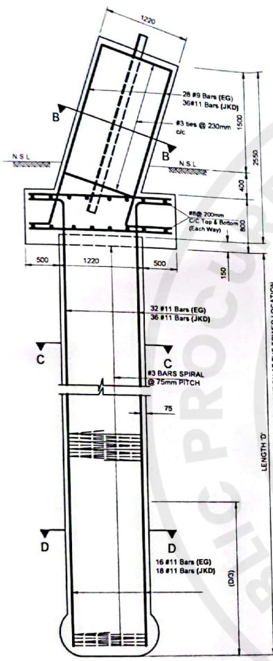
SECTION A-A
