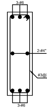
B-2 (END SPAN) (9"x 30")
