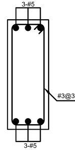
B-1 (END SPAN) (9"x 24")
